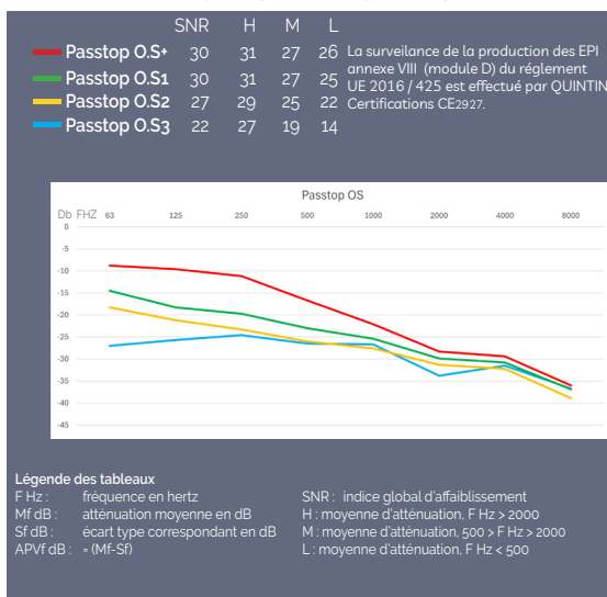
COURBES D'ATTENUATIONS
